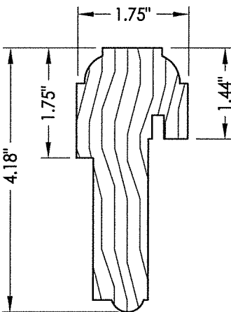
35 ASTRAGAL
